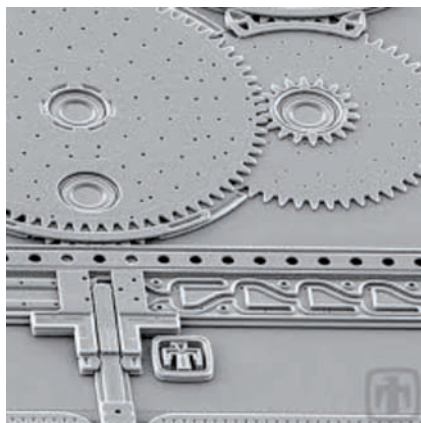
Figura 13. Nanoengranaje fabricado mediante técnica top-down .
